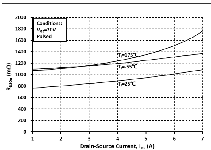
图. 6 各温度下的 R_{on} 和 I_{DS} 关系曲线
