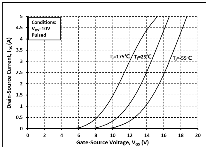
图. 8 各温度下的传输特性曲线
