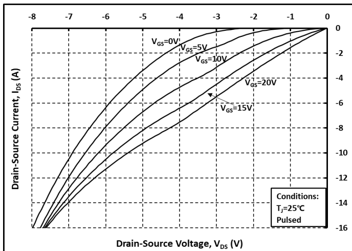
图. 14 第三象限曲线 @ T_j = 25^\circ\text{C}
