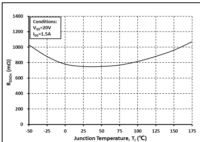
图. 4 R_{on} 和温度关系曲线
