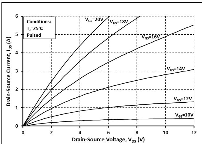
图. 2 输出曲线 @ T_j = 25^\circ\text{C}
