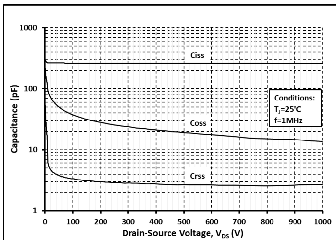
图. 16 各电容和 V_{DS} 关系曲线
